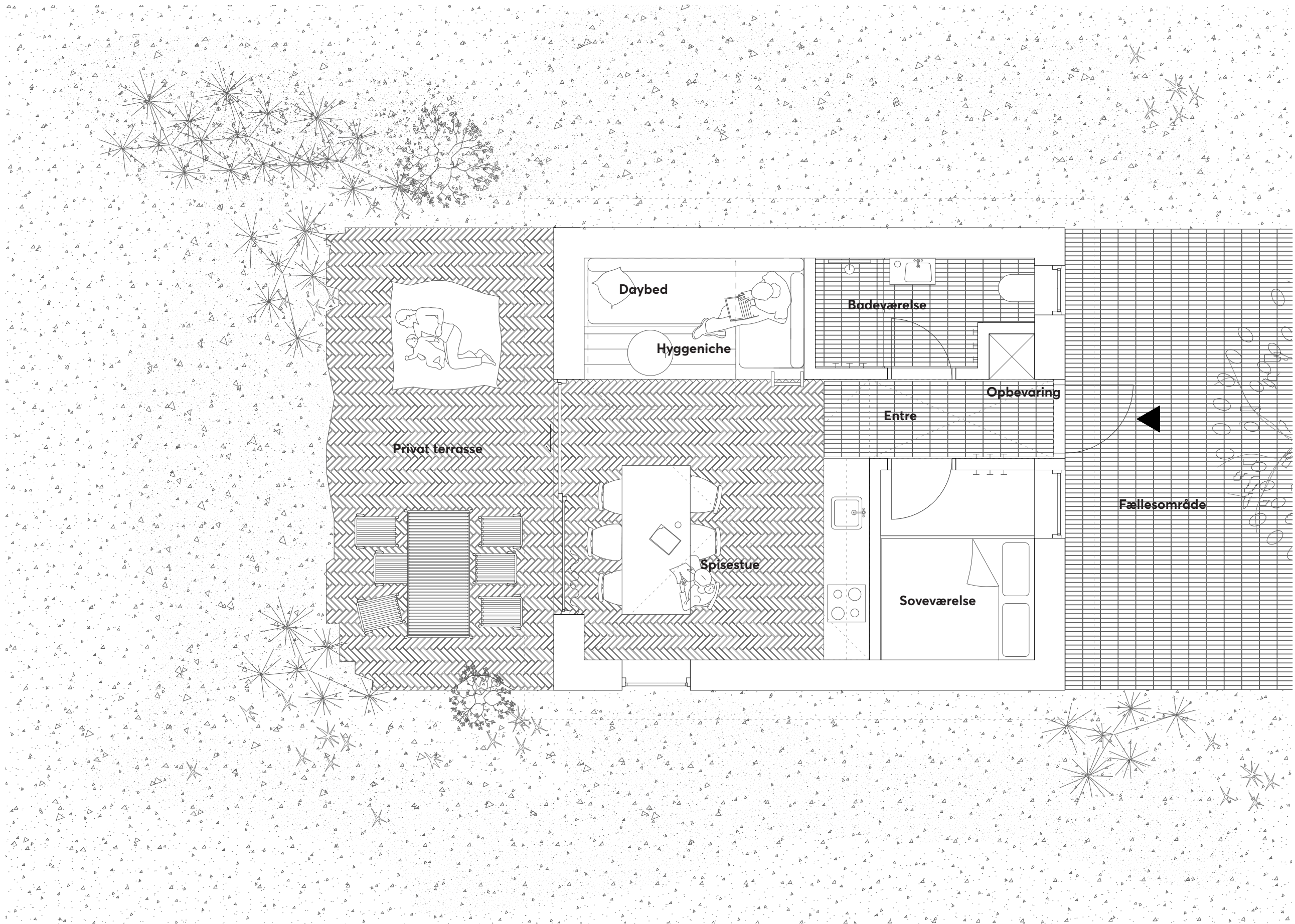
Plan 1:50
